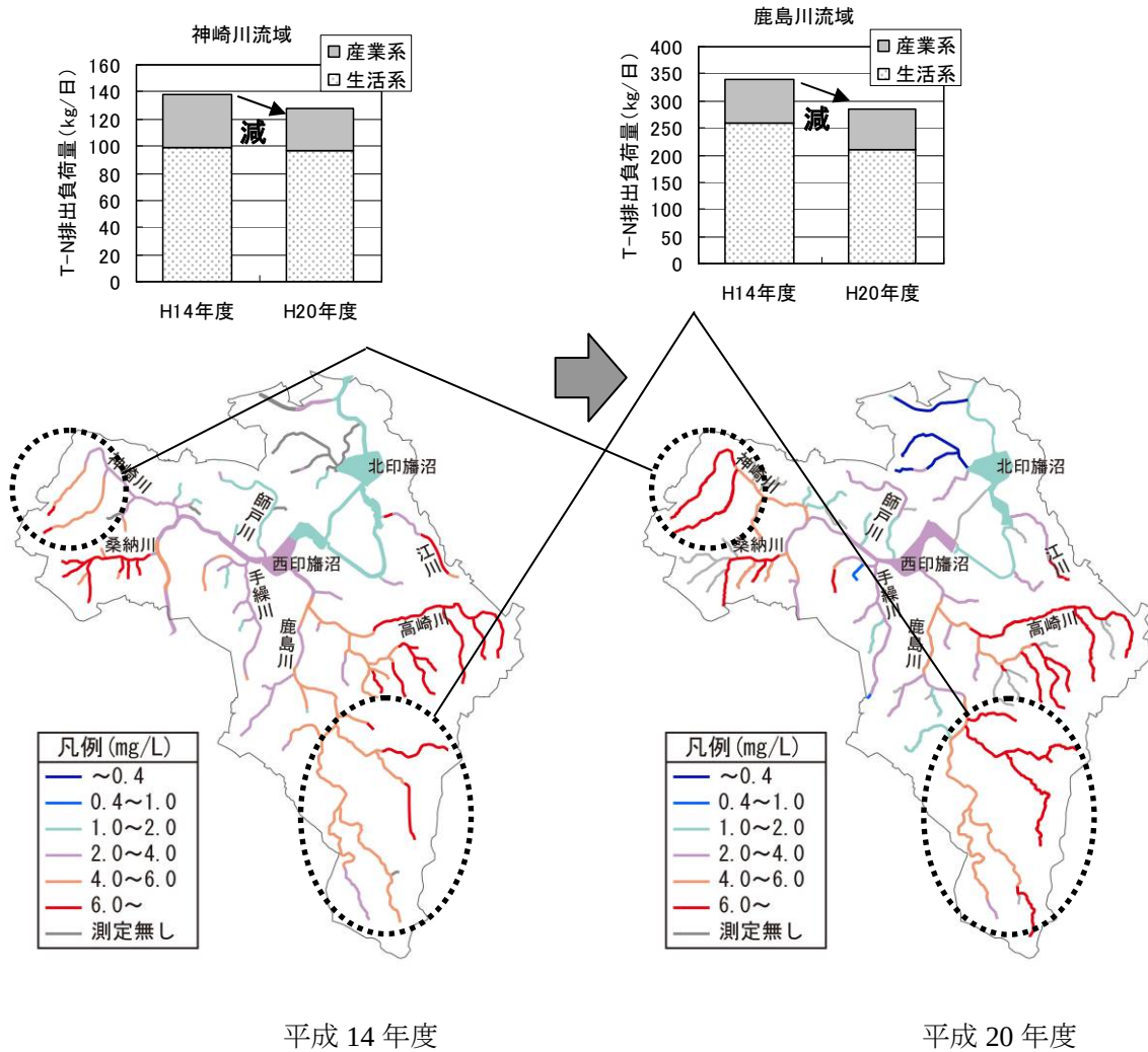
図 2.20 河川水質 T-N 年平均值の変化と排出負荷量の比較
