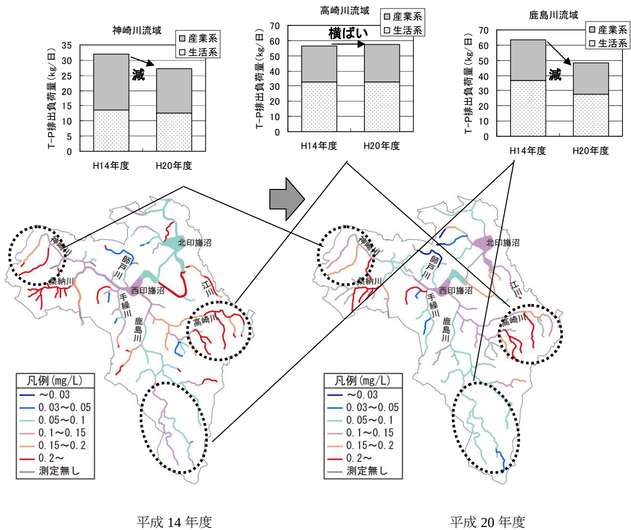
図 2.21 河川水質 T-P 年平均值の変化と排出負荷量の比較
